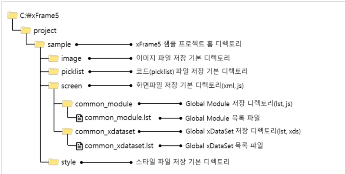
그림. 샘플 디렉토리 구조
